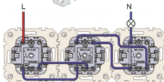
Łącznik krzyżowy w układzie z dwoma łącznikami schodowymi.
