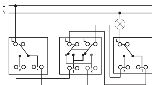
Schemat podłączenia łącznika krzyżowego w układzie z dwoma łącznikami schodowymi.
